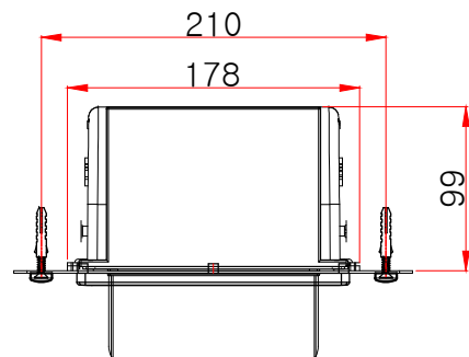
평(상)면도
