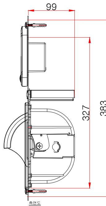
측면도
