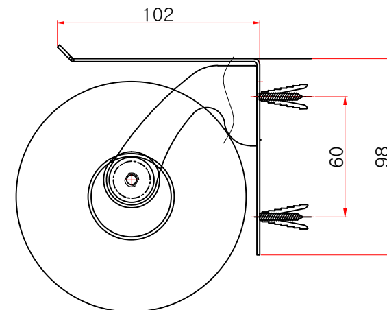
우측면도
