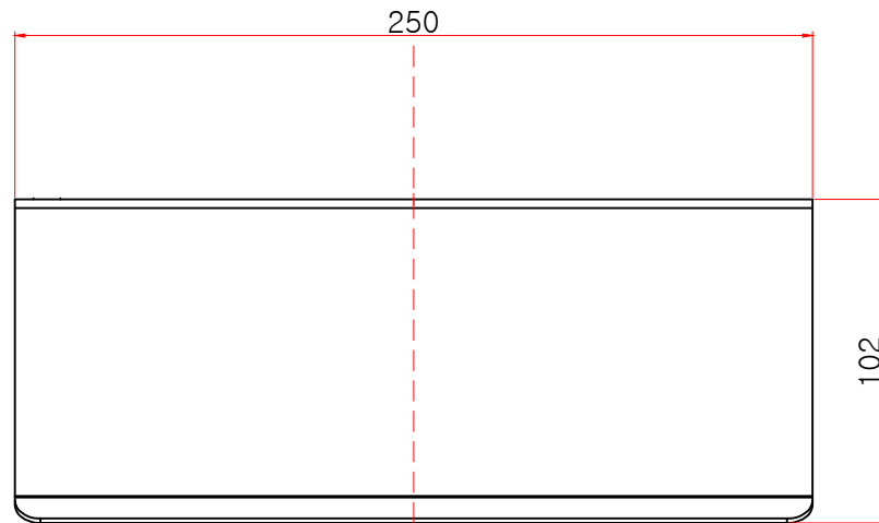
평(윗)면도
