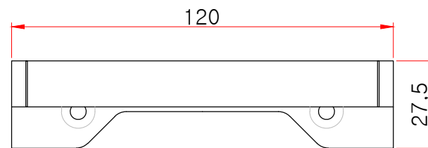
정면도
