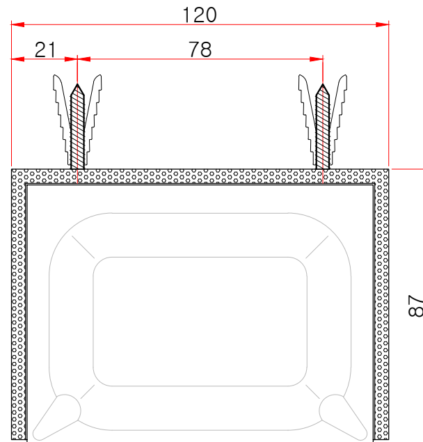
평(윗)면도
