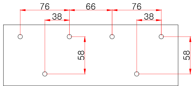
배(후)면도 (피스hole-center)
