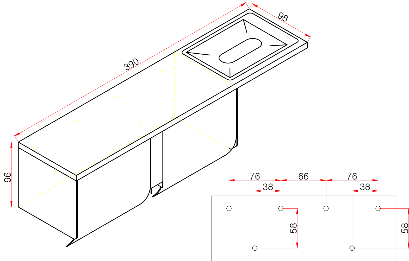
배(후)면도 (피스hole-center)
