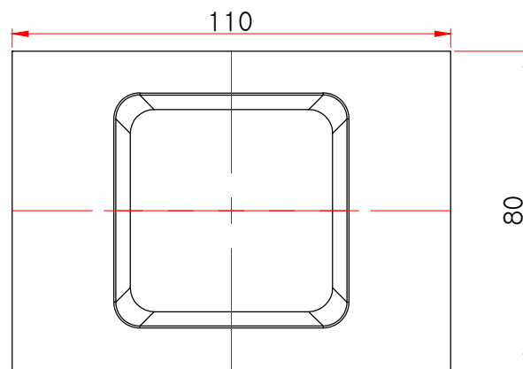
평(윗)면도
