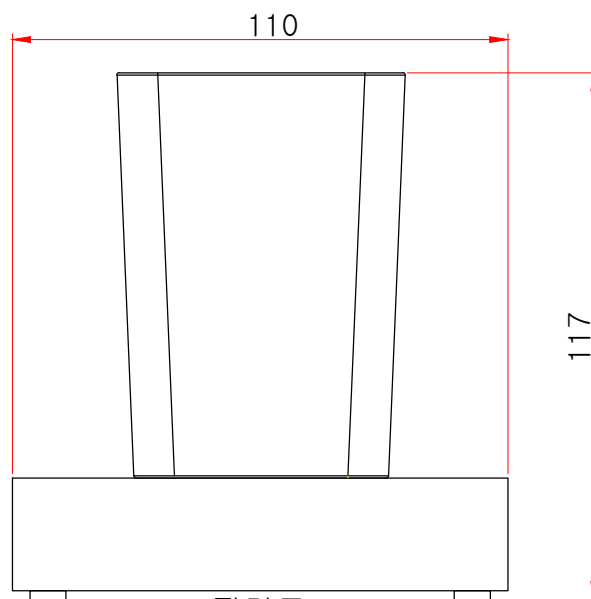
정면도
