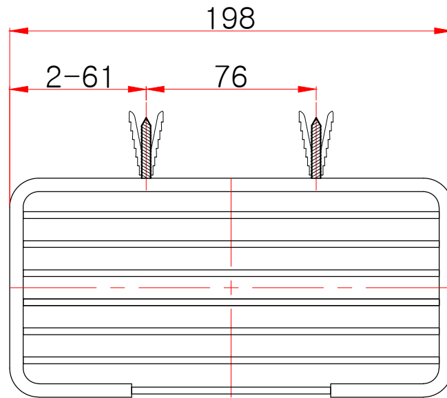
평(윗)면도
