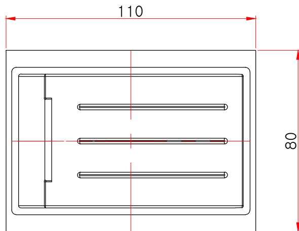
평(윗)면도
