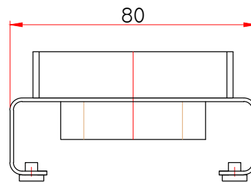
측면도
