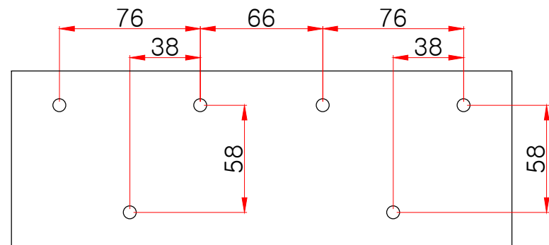
배(후)면도 (피스hole-center)
