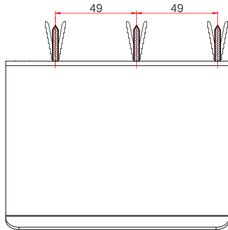
평(윗)면도
