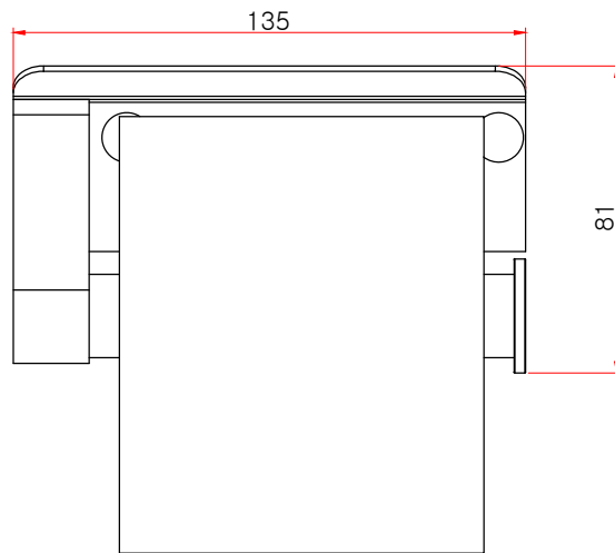
정면도
