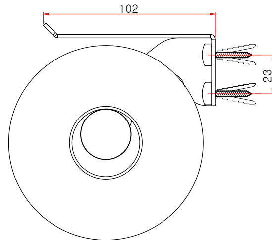
우측면도
