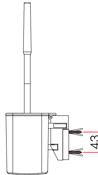
측면도
