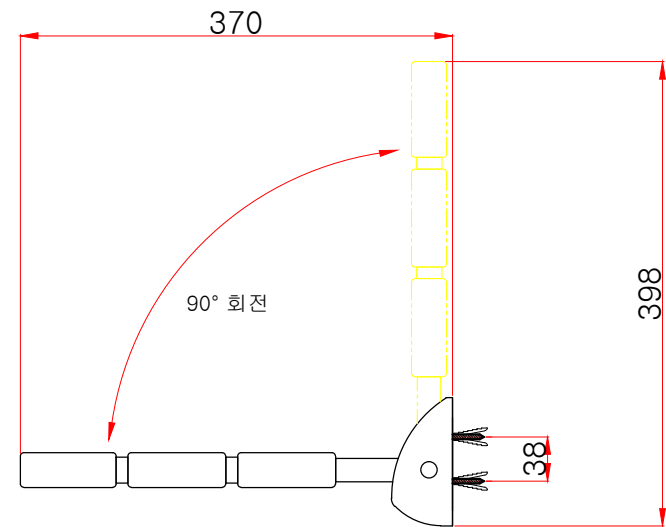
측면도
