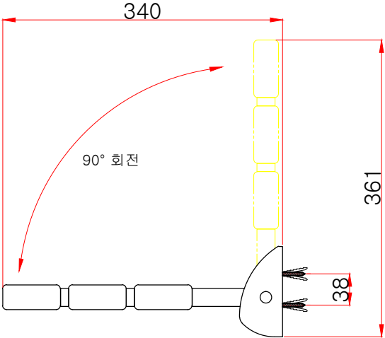
측면도
