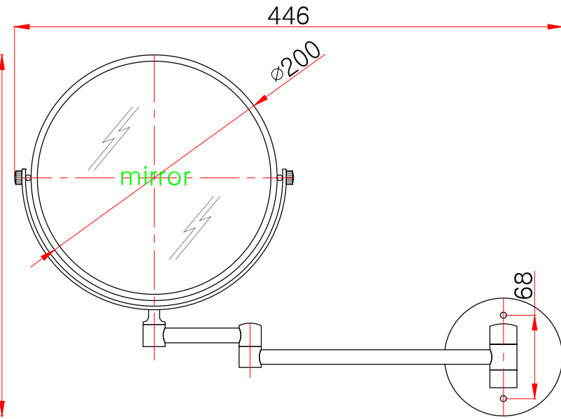
정면도
