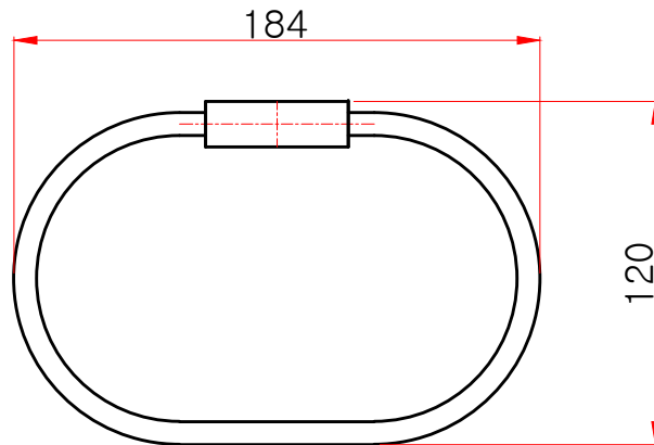
정면도
