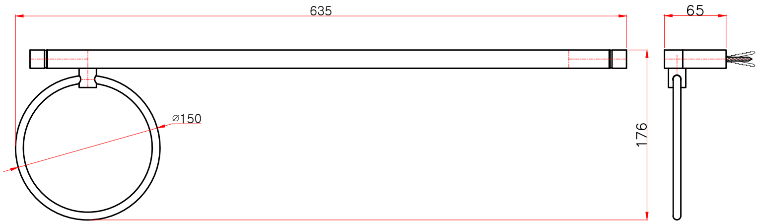
정면도
