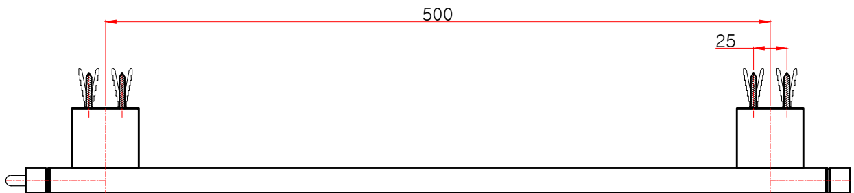
평(윗)면도
