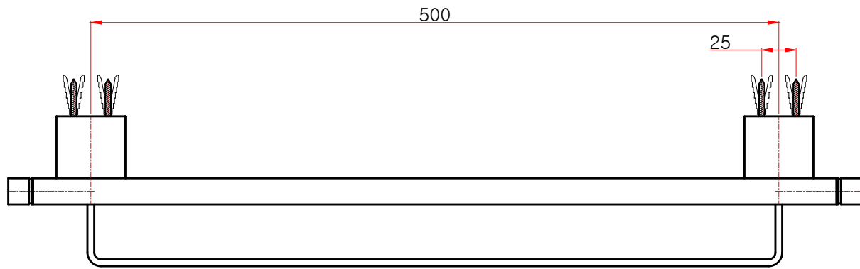
평(윗)면도
