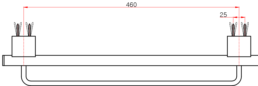
평(윗)면도
