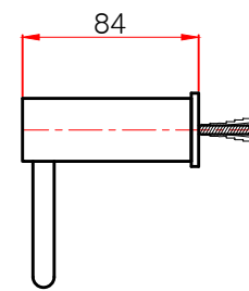
측면도
