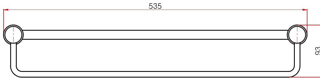
정면도
