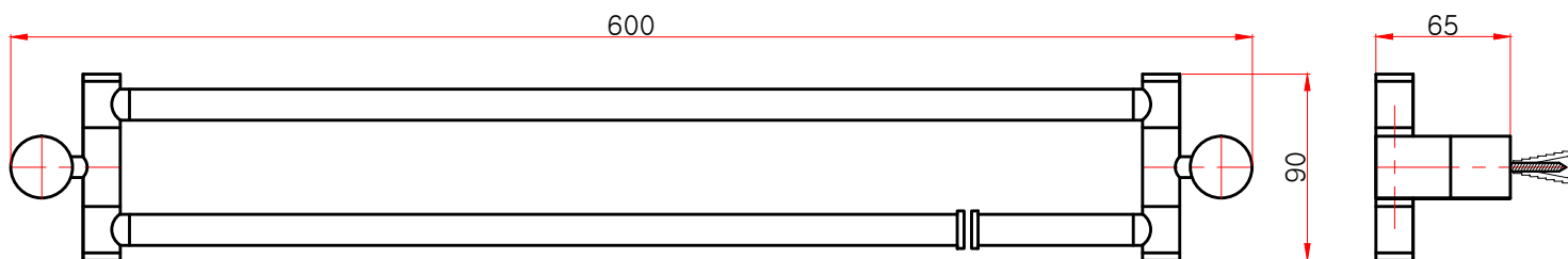
정면도
