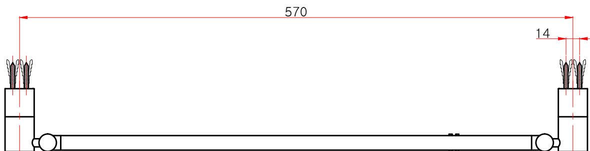
평(윗)면도
