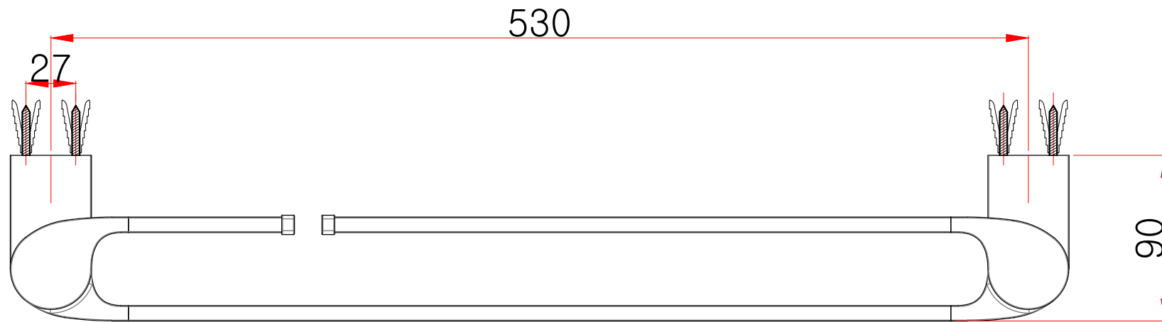
평(윗)면도
