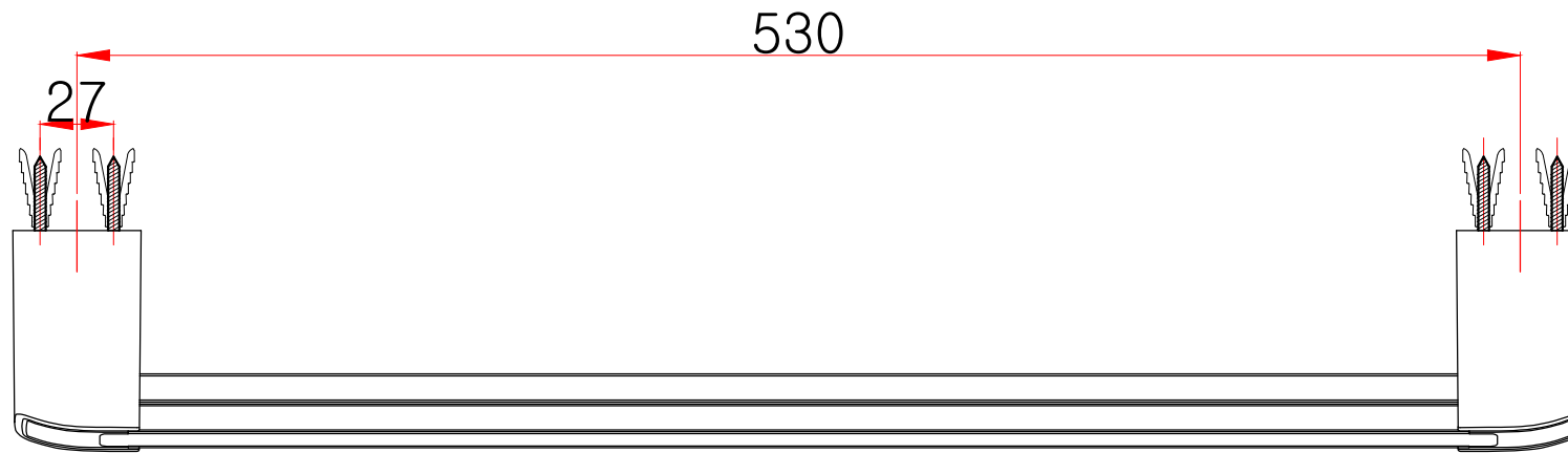
평(윗)면도
