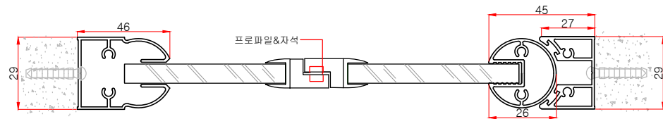
Detail A - A'
