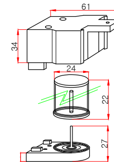
도어캡 - C -
