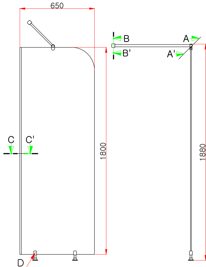
정면도
