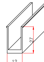
U-채널(벽) C - C'
