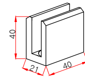
사각클립 40*40 - E -
