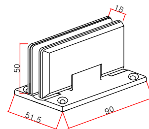
경첩 - B -
