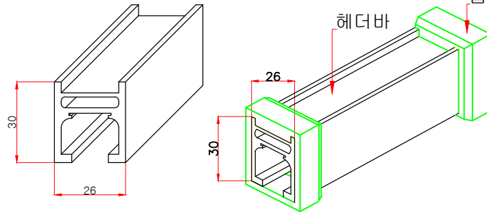
사각헤더바 A - A'
