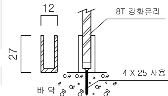
U-채널(바닥) E - E'
