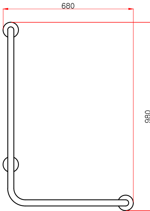
정면도
