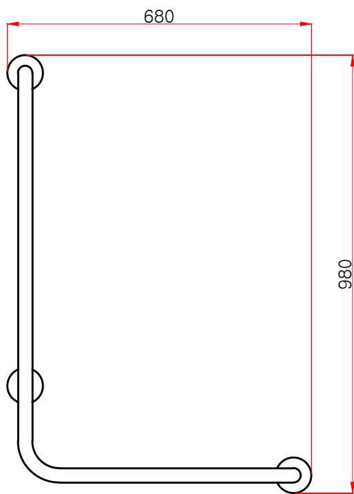
정면도
