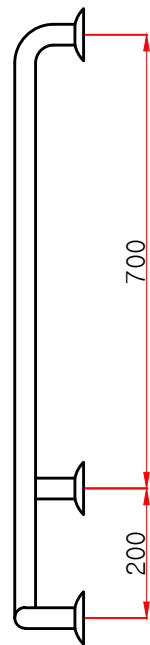
측면도
