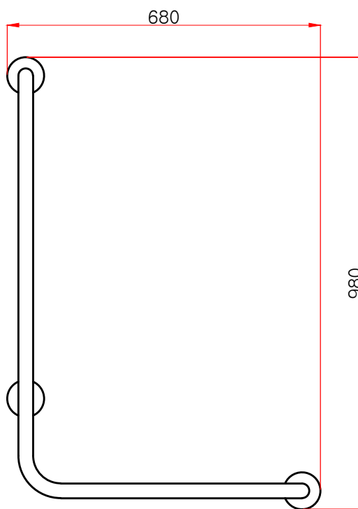
정면도
