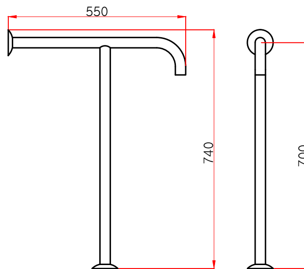
정면도
