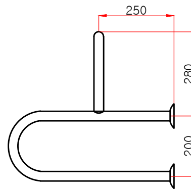
측면도
