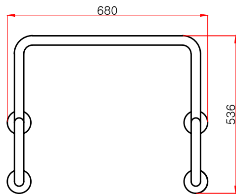
정면도
