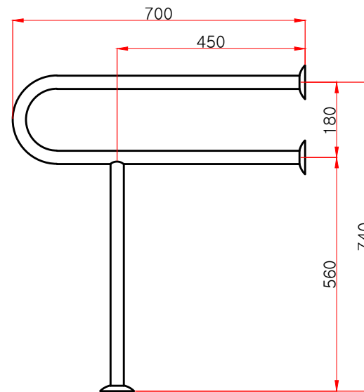
측면도
