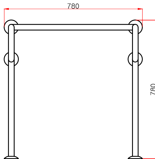
정면도
