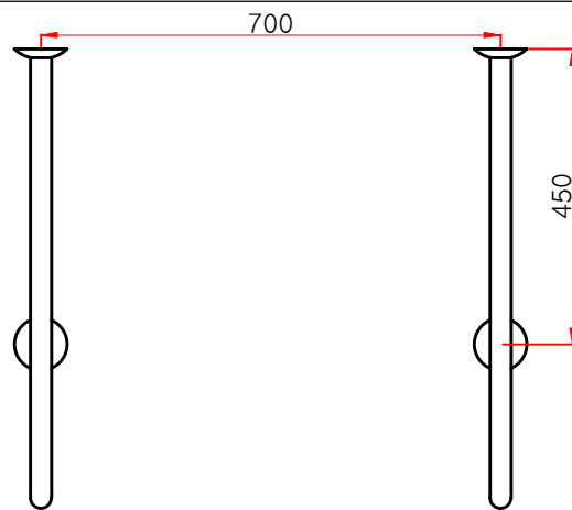
평(윗)면도
