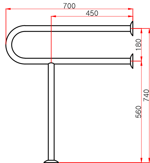
측면도
