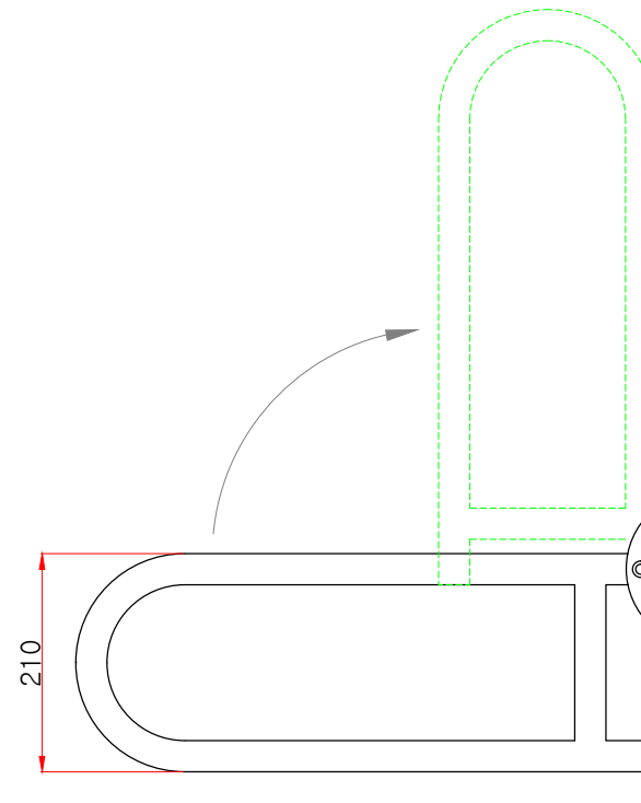
측면도
