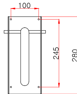
정면도
