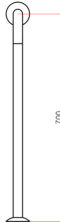
측면도
