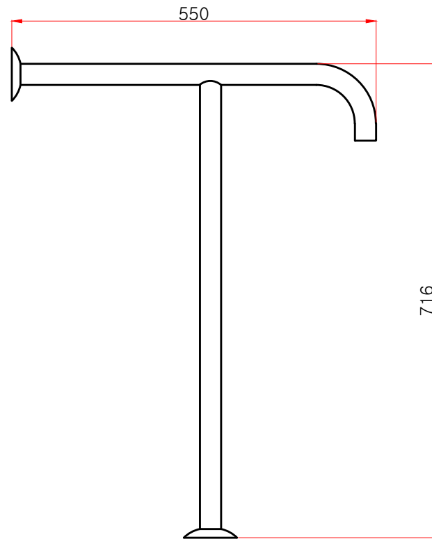
정면도
