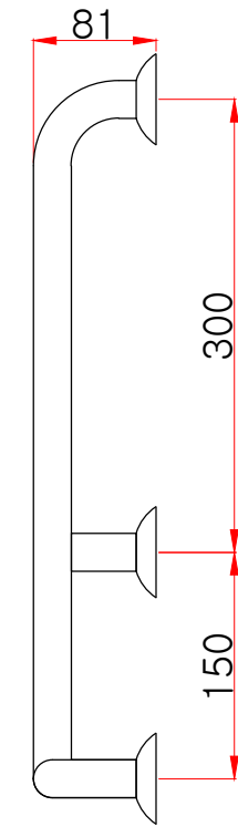
측면도
