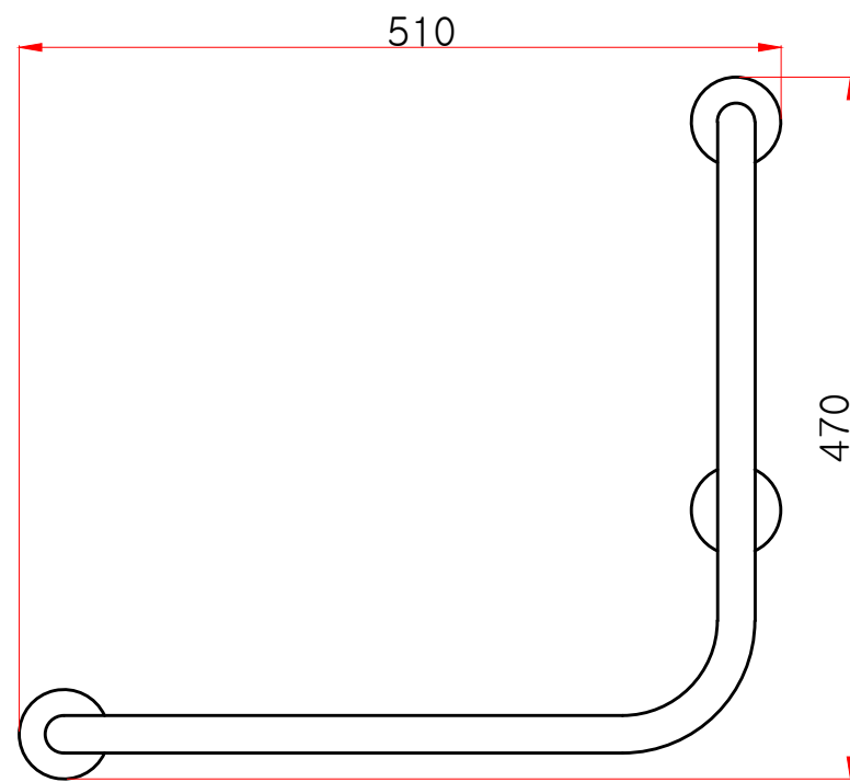
정면도
