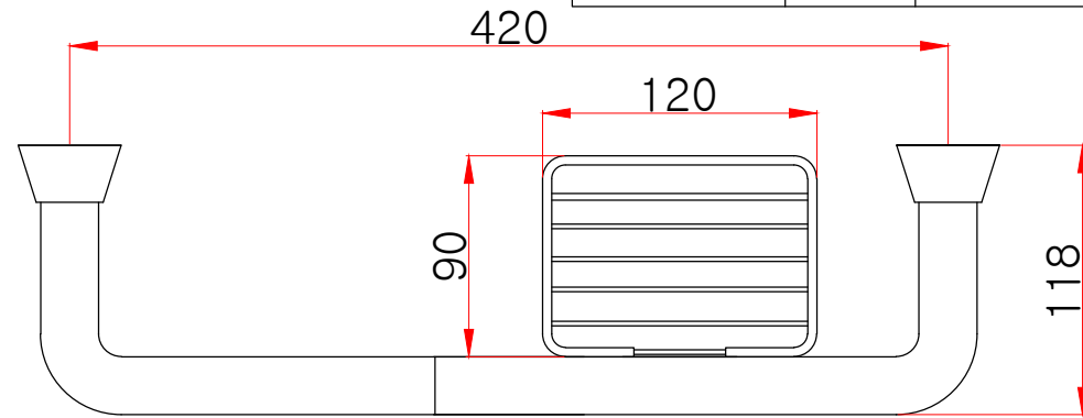
평(윗)면도
