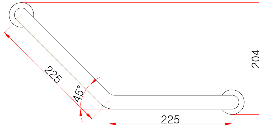
정면도
