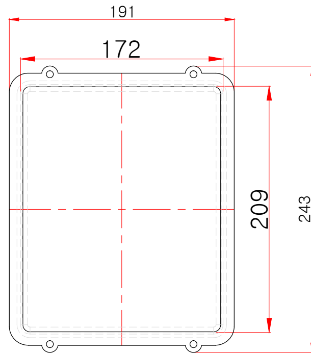
정면도
