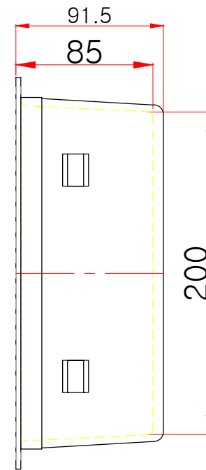
측면도
