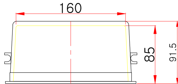
평(윗)면도
