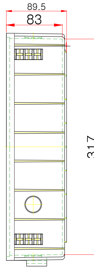
측면도
