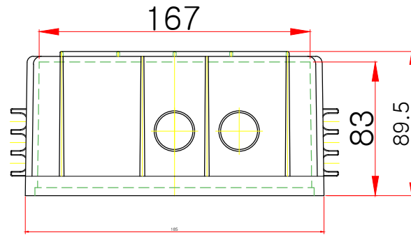
평(윗)면도
