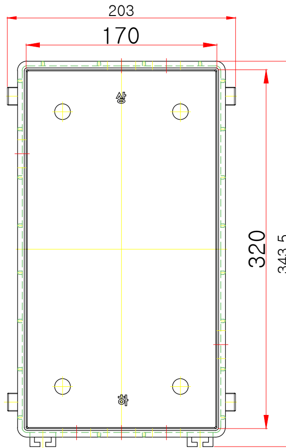
정면도
