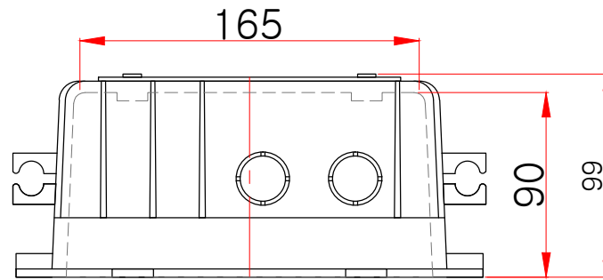
평(윗)면도
