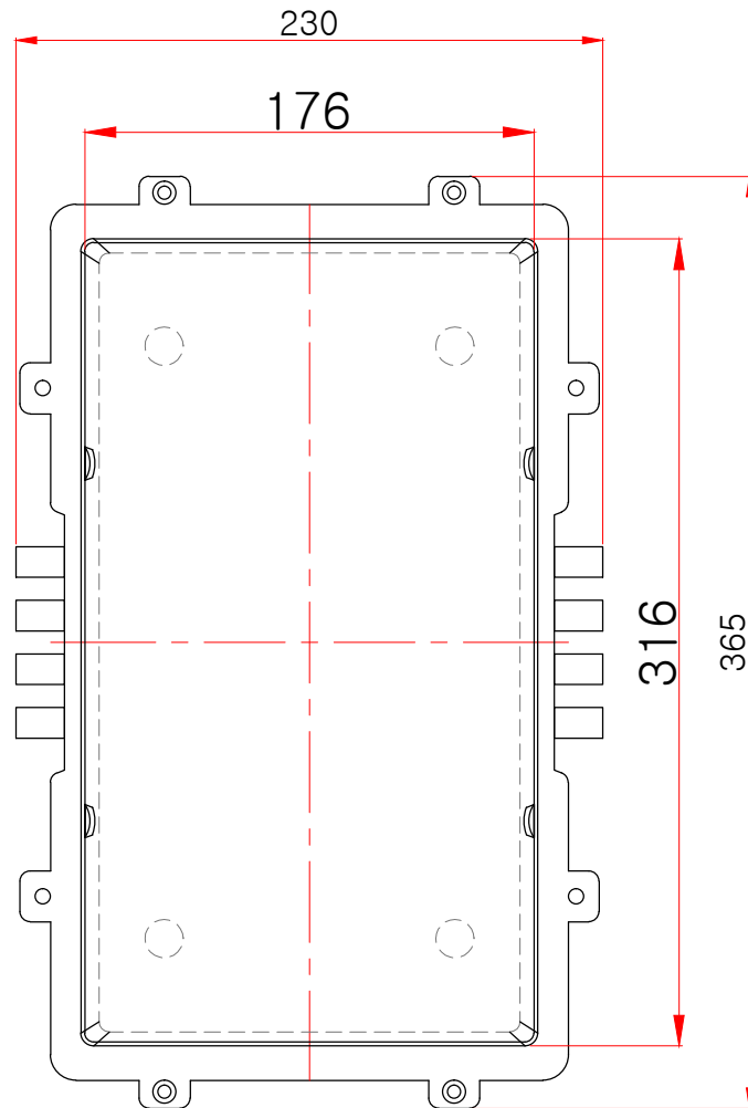
정면도
