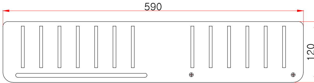
평(윗)면도
