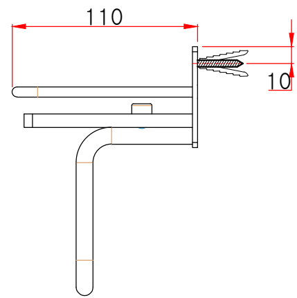
측면도
