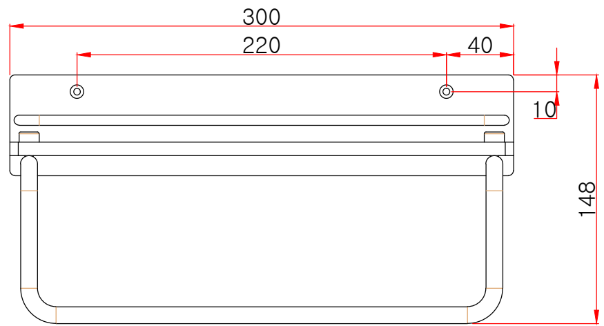
정면도
