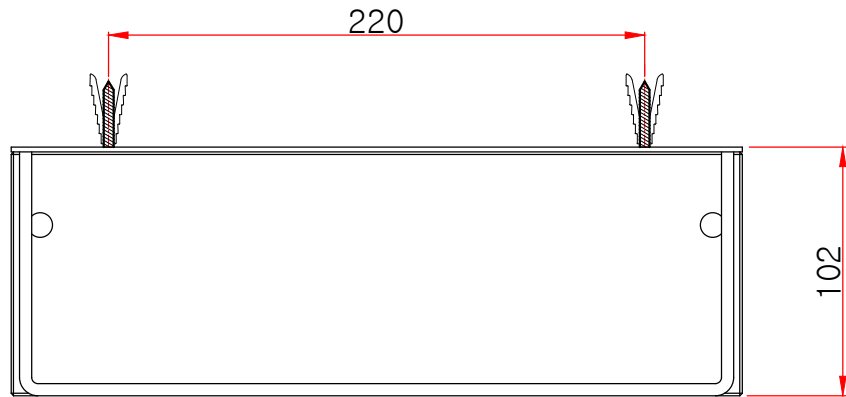
평(윗)면도
