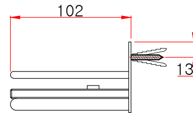
측면도
