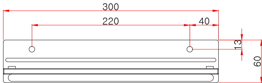
정면도
