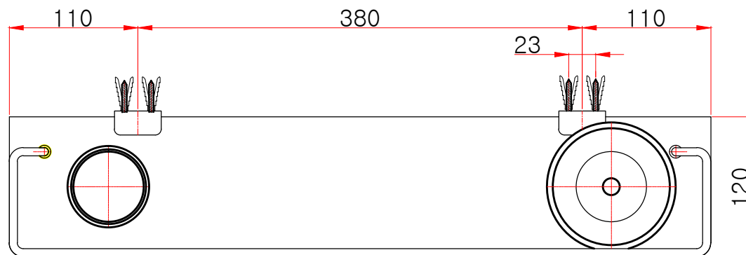
평(위)면도
