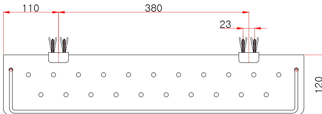
평(윗)면도
