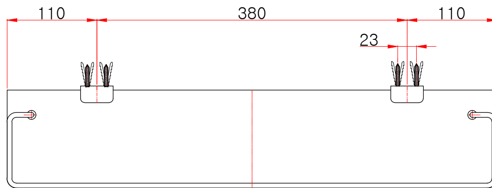
평(윗)면도
