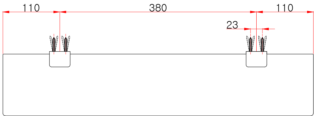
평(윗)면도
