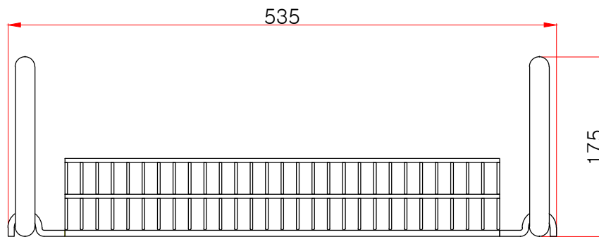
정면도
