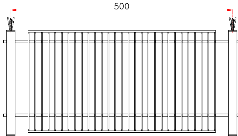
평(위)면도
