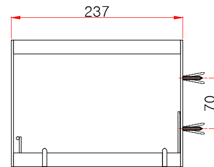
측면도
