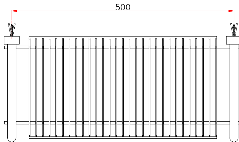
평(윗)면도
