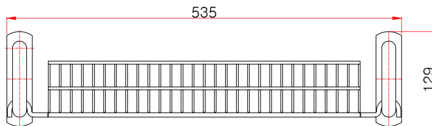
정면도
