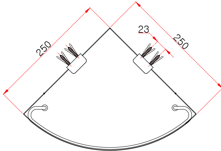
평(윗)면도
