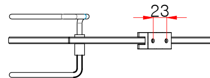
측면도
